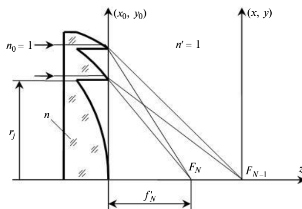
Рис. 2. Визначення БПДЛ і фокальних точок різних порядків
