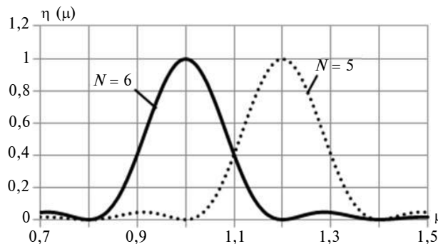
Рис. 7. Дифракційна ефективність для різних порядків дифракції
