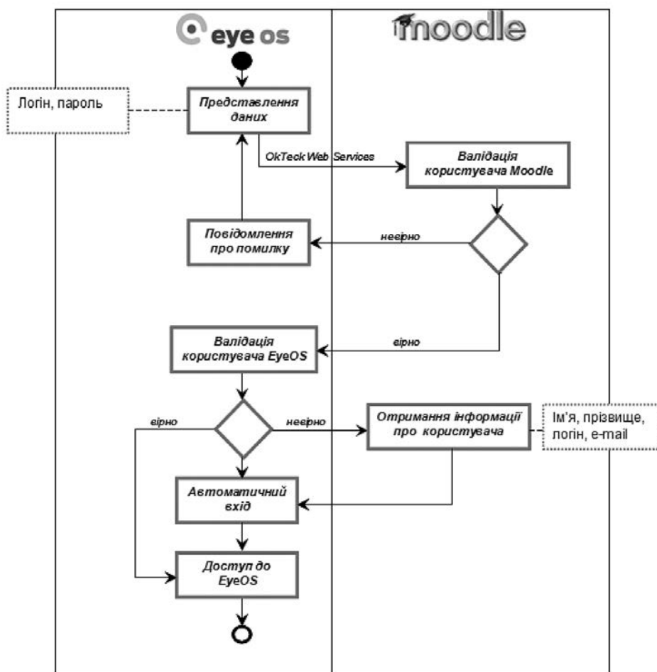
Рис. 2. Архітектура Moodle
