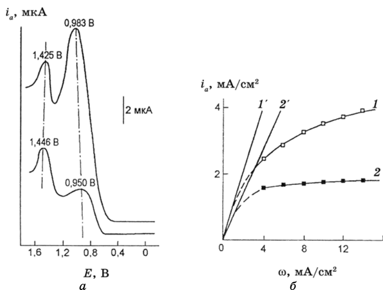
Рис. 2. Зависимость величины анодного пика электроокисления тиокарбамида при концентрации C_{TK} = 2,81 \cdot 10^{-3} М (1) и C_{TK} = 5,62 \cdot 10^{-3} М (2) от потенциала стеклоуглеродного электрода (а); зависимость анодного тока золота в максимуме (1) и минимуме (2) вольтамперной кривой от скорости вращения электрода \omega по [6], дополненная нашими данными (1' и 2') (б).
