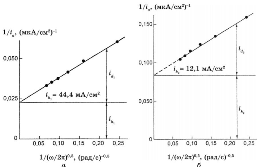
Рис. 3. Зависимость обратной величины анодных токов максимумов ( 1/i_a ) вольтамперной кривой от обратной скорости вращения электрода ( 1/(\omega/2\pi)^{1/2} ); где i_{k_i} — кинетические токи. а) [Au(I)] = 0,0152 М, C_{TK} = 2,81 \cdot 10^{-3} М; б) [Au(I)] = 0,0152 М, C_{TK} = 5,62 \cdot 10^{-3} М.
