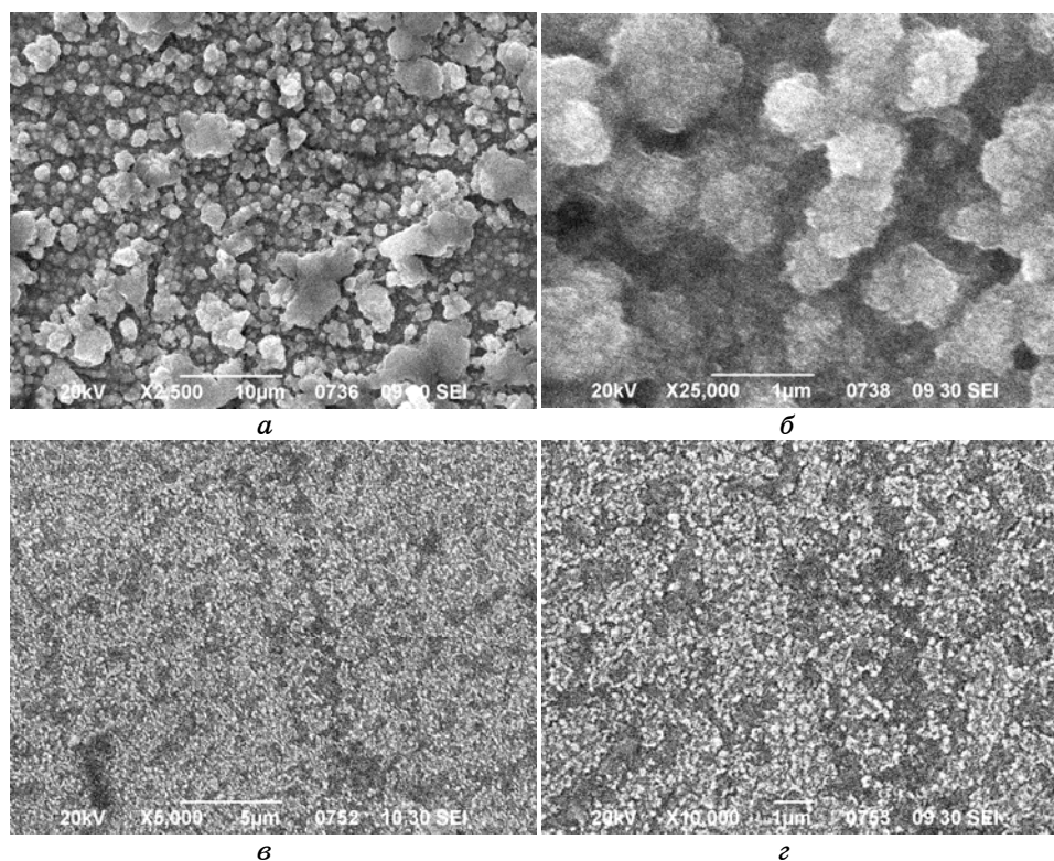
Рис. 4. Растровая электронная микроскопия нанодисперсного сферидного золота, осаждённого на Ni-электроде из двухфазной водно-органической системы толуол-водный раствор 0,1 \text{ M } (\text{NH}_2)_2\text{CS} + 0,005 \text{ M H AuCl}_4 + 0,01 \text{ M C}_2\text{H}_4(\text{COOH})_2 + 0,01 \text{ M C}_3\text{H}_4(\text{OH})(\text{COOH})_3 при объёмном соотношении органическая фаза-водный раствор 1:5 с 3 об.% этанола при плотности тока i_k = 2 \text{ A/дм}^2 , времени электролиза \tau = 6 мин и температуре 30^\circ\text{C} . Увеличение 5000 (а). (б) — то же при увеличении 25000; (в) — то же при плотности тока 10 \text{ A/дм}^2 и увеличении 5000; г — то же при увеличении 10000.
