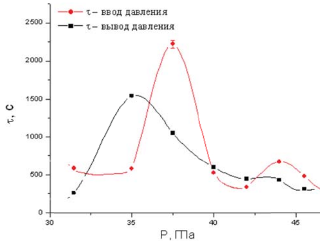
Рис. 4. Барические зависимости характерного времени релаксации для образца ZrO_2 с размерами кристаллитов 12 нм при повышении и снижении давления.
