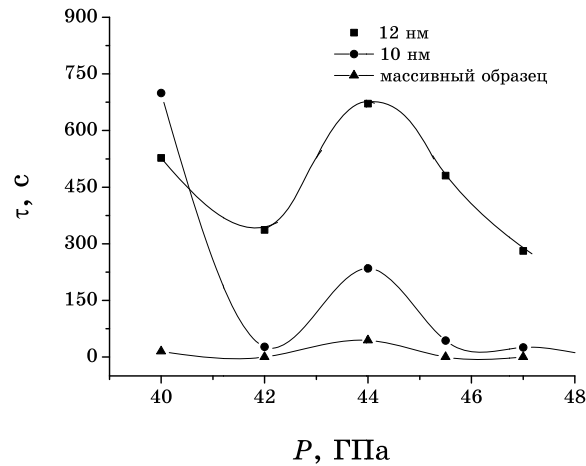
Рис. 5. Барические зависимости характерного времени релаксации для образцов ZrO_2 с размерами кристаллитов 10 и 12 нм и для массивного образца.
