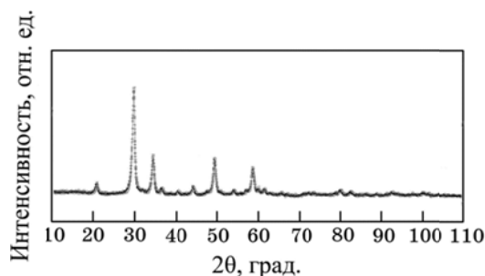
Рис. 7. Рентгенограмма оксида лютетия, полученного при низкотемпературной кристаллизации прекурсора ( T = 1000^\circ\text{C} ).
