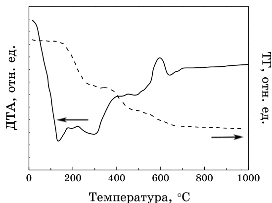
Рис. 5. ДТА–ТГ-кривая процесса термического разложения кристаллического прекурсора оксида лутеция.
