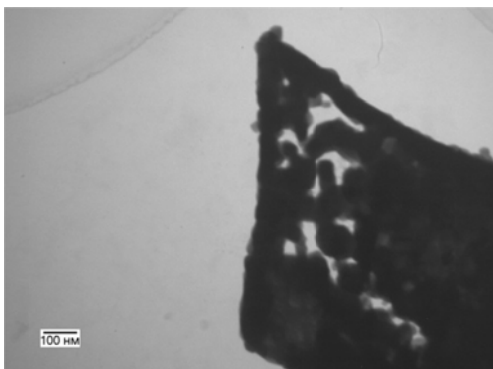
Рис. 6. ПЭМ-изображения частиц оксида лутеция, полученных при низкотемпературной кристаллизации прекурсора при T = 1000^\circ\text{C} .
