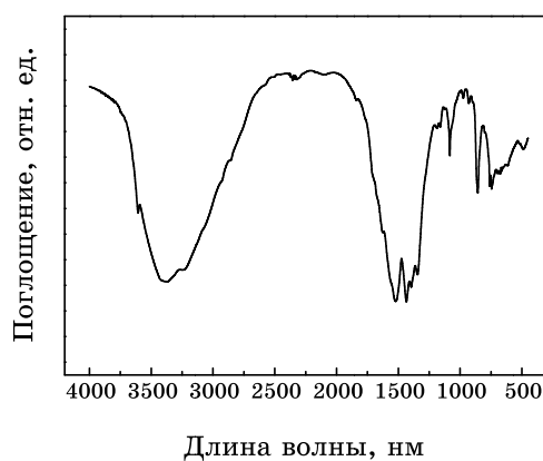
Рис. 4. ИК-спектры прекурсора оксида лутеция, полученного при R = 8-20 .
