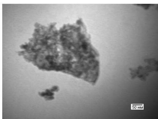
Рис. 2. ПЭМ-изображения частиц прекурсора оксида лутеция, полученного при R = 8-20 , времени старения 24 ч. и температуре 25°C.
