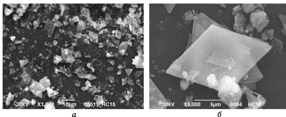
Рис. 1. СЭМ-изображения частиц прекурсора оксида лутеция, полученного при R = 8-20 , времени старения 24 ч. и температуре 25°C.
