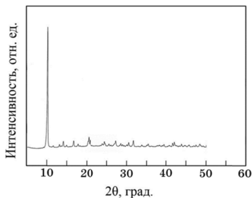
Рис. 3. Рентгенограммы карбонатного прекурсора оксида лутеция, полученного при R = 8-20 .
