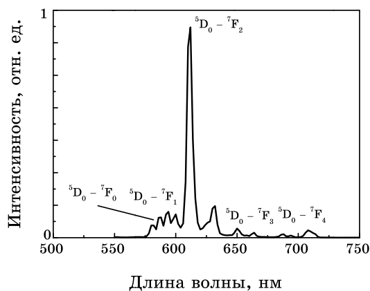
Рис. 8. Спектр радиолюминесценции \text{Lu}_2\text{O}_3:\text{Eu}^{3+} (5 ат.%).
