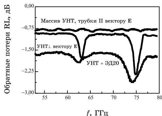
Рис. 6. Частотные зависимости обратных потерь для массива ориентированных нанотрубок (при различных ориентациях нанотрубок относительно вектора электрического поля ЭМИ) и эпоксидного композита с изотропно распределенными диспергированными фрагментами массива многослойных нанотрубок, размер образцов 3,6 \times 1,8 \times 1,0 мм 3 .
