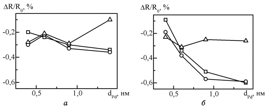
Рис. 4. Зависимость магнитосопротивления от толщины Pd для системы [\text{Pd}(x)/\text{Fe}(0,6)]_{10}/\Pi при T = 300 К (а) и после отжига до 780 К (б).
