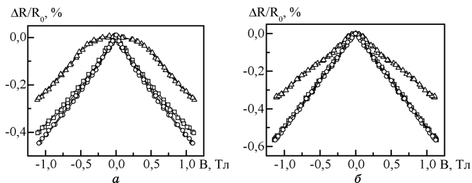
Рис. 5. Зависимость МС для [\text{Cu}(0,2)/\text{Fe}(0,9)/\text{Pd}(1,1)]_5/\Pi при T = 300 К (а) и после отжига до 780 К (б).
