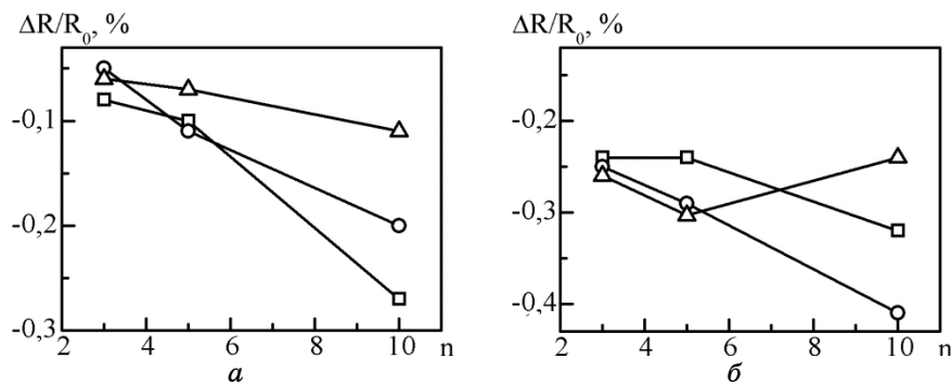
Рис. 3. Зависимость МС от количества повторяемости слоев n для системы [\text{Pd}(1,1)/\text{Fe}(0,9)]_n/\text{П} при T = 300 \text{ К} (а) и после отжига до 780 \text{ К} (б).
