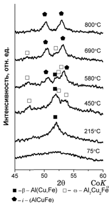
Рис. 3. Рентгеновские дифрактограммы, снятые в процессе непрерывного нагрева вакуумного конденсата Al_{63}Cu_{26}Fe_{11} , осажденного при температуре подложки 250–300°C.
