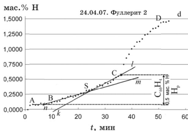
Рис. 11. Адсорбция H_2 и двухстадийная абсорбция водорода в ГЦК-решетке фуллерита. Стрелкой отмечено содержание решеточного водорода ( H_p ).
