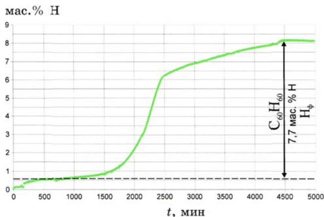
Рис. 12. Экспериментальная кривая взаимодействия газообразного водорода с фуллеритом. Стрелкой отмечена доля фуллерированного водорода ( H_{\Phi} ).
