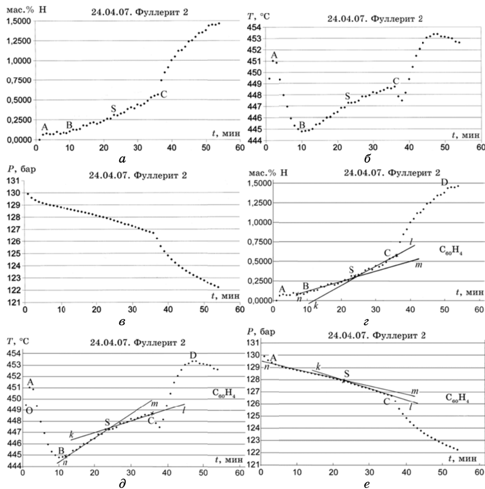
Рис. 6. Экспериментальные зависимости, полученные в результате исследования взаимодействия водорода с фуллеритом, отражающие образование твердого раствора водорода в фуллерите: a , z — зависимость изменения массы фуллерита во времени; б , д — изменение температуры фуллерита во времени; в , е — изменение давления водорода в реакторе. Расстояние между точками на диаграммных кривых соответствует одной минуте. Рисунки z , д , е дополнены вспомогательными линиями « nt » и « kl ». Участок «BS» соответствует абсорбции молекулярного водорода, «SC» — соответствует диссоциативной абсорбции водорода.
