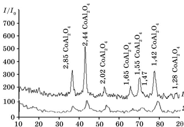
Рис. 5. Рентгенівська дифрактограма пігменту, який був одержаний співосадженням з сульфатів алюмінію та кобальту, із \text{CuK}_\alpha -випроміненням: 1 — вагове співвідношення \text{Co}:\text{Al} = 2:1 , 2 — співвідношення \text{Co}:\text{Al} = 1:2 .
