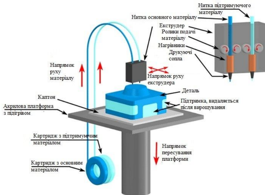
Рис. 1. Схематичне зображення роботи 3D-принтера
