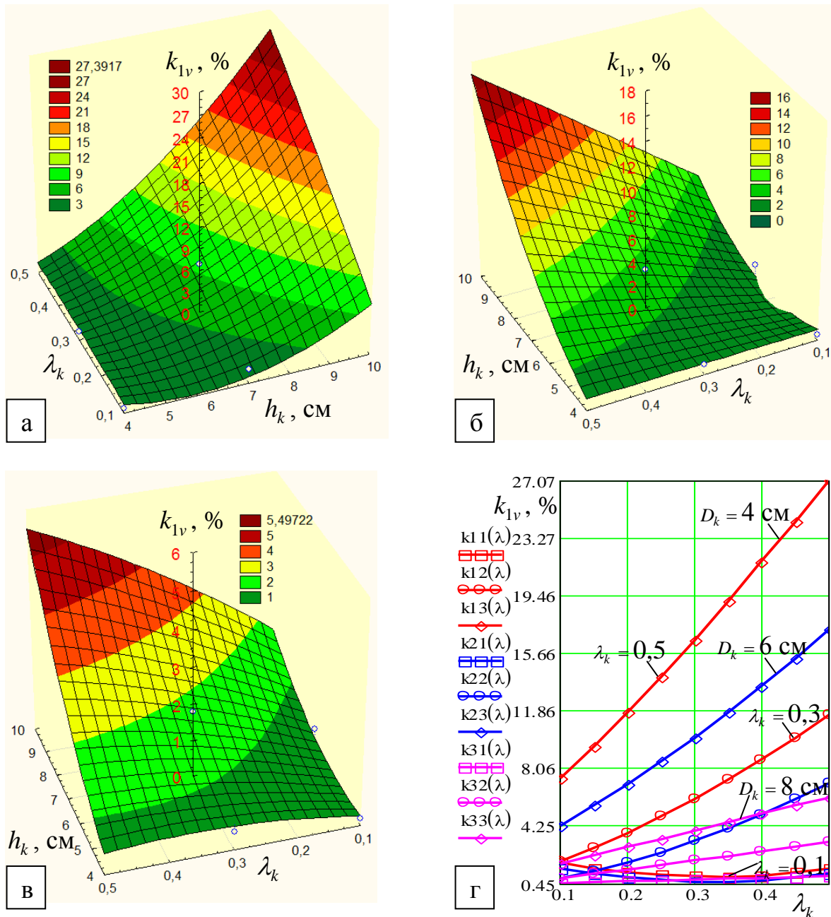
Рис. 5. Поверхня відгуку зміни k_{lv}^{(i)} за умови \alpha_z = 0 :
