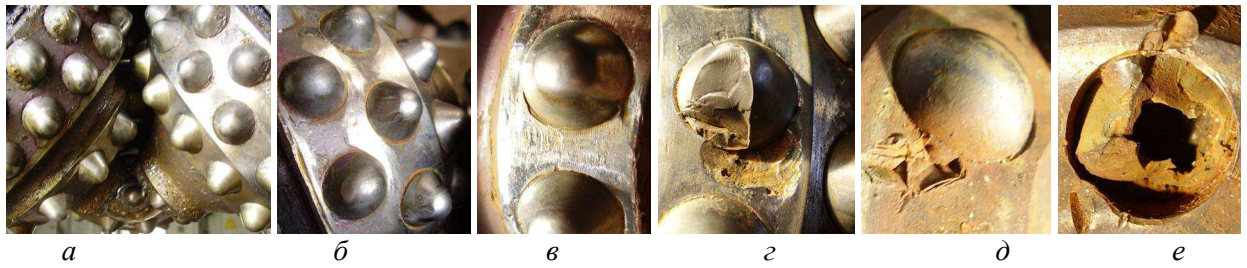
а – 13 годин роботи долота (загальний вигляд піднесено над вибоєм долота) ; б – 20 годин роботи долота (ділянка вінця шарошки секції № 3 ; в – 24 годин роботи долота (ділянка вінця шарошки секції № 2); г – 24 години роботи долота (ділянка вінця шарошки секції № 3); д – 24 годин роботи долота (ділянка вершини шарошки секції № 3); е – 30 годин роботи долота (ділянка вершини шарошки секції № 3)
