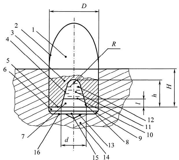
1 – твердосплавний елемент, 2 – робоча головка, 3 – хвостовик, 4 – порожнина хвостовика, 5 – торець хвостовика, 6 – диск, 7 – зрізаний конус, 8 – конічна поверхня, 9 – західна фаска, 10 – площина зрізаного конуса, 11 – камера, 12 – гліцерин, 13 – конічна заглибина, 14 – тіло породоруйнівного інструменту (шарошка долота), 15 – основа диска, 16 – дно отвору в шарошці
