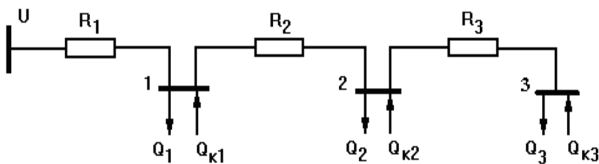
Рисунок 9 – Схема електропостачання
