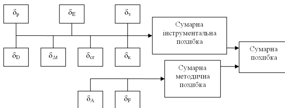
Рисунок 4 – Схема накопичення сумарної похибки вимірювального каналу тиску САК за відборами нафти з МН
