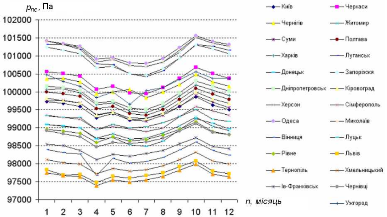
Рисунок 1 – Зміна фактичних середньомісячних значень атмосферного тиску в обласних центрах України
