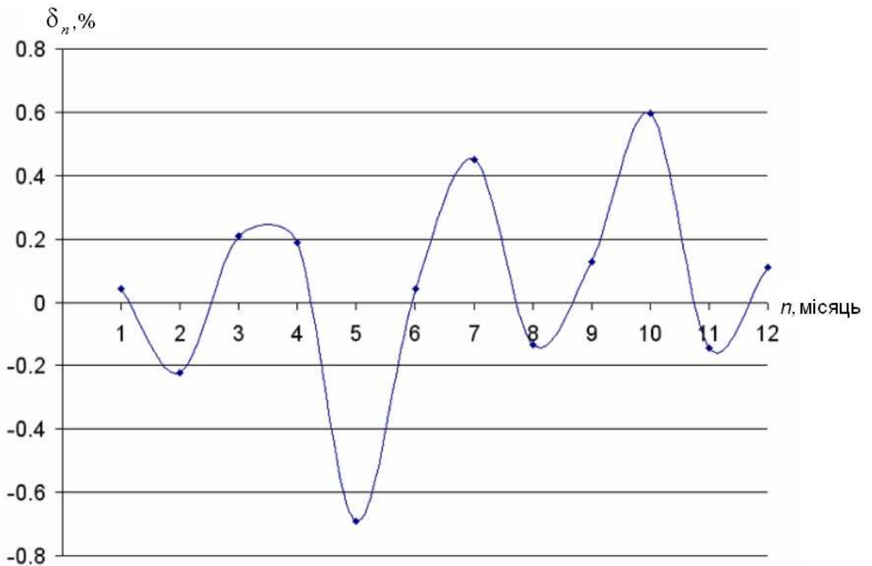
Рисунок 5 – Похибки виміряних і змодельованих значень атмосферного тиску в м. Києві в 2010 р.
