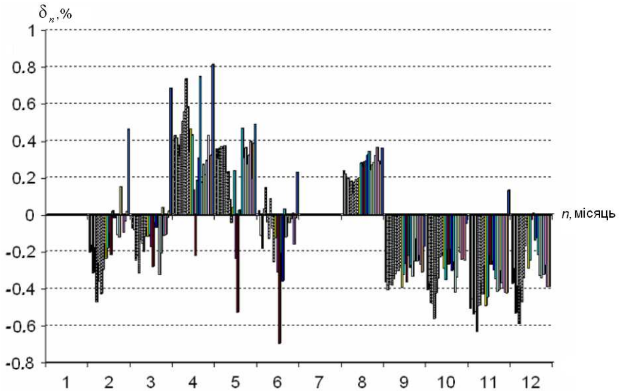
Рисунок 4 – Відносна похибка вимірних і обчислених значень атмосферного тиску
