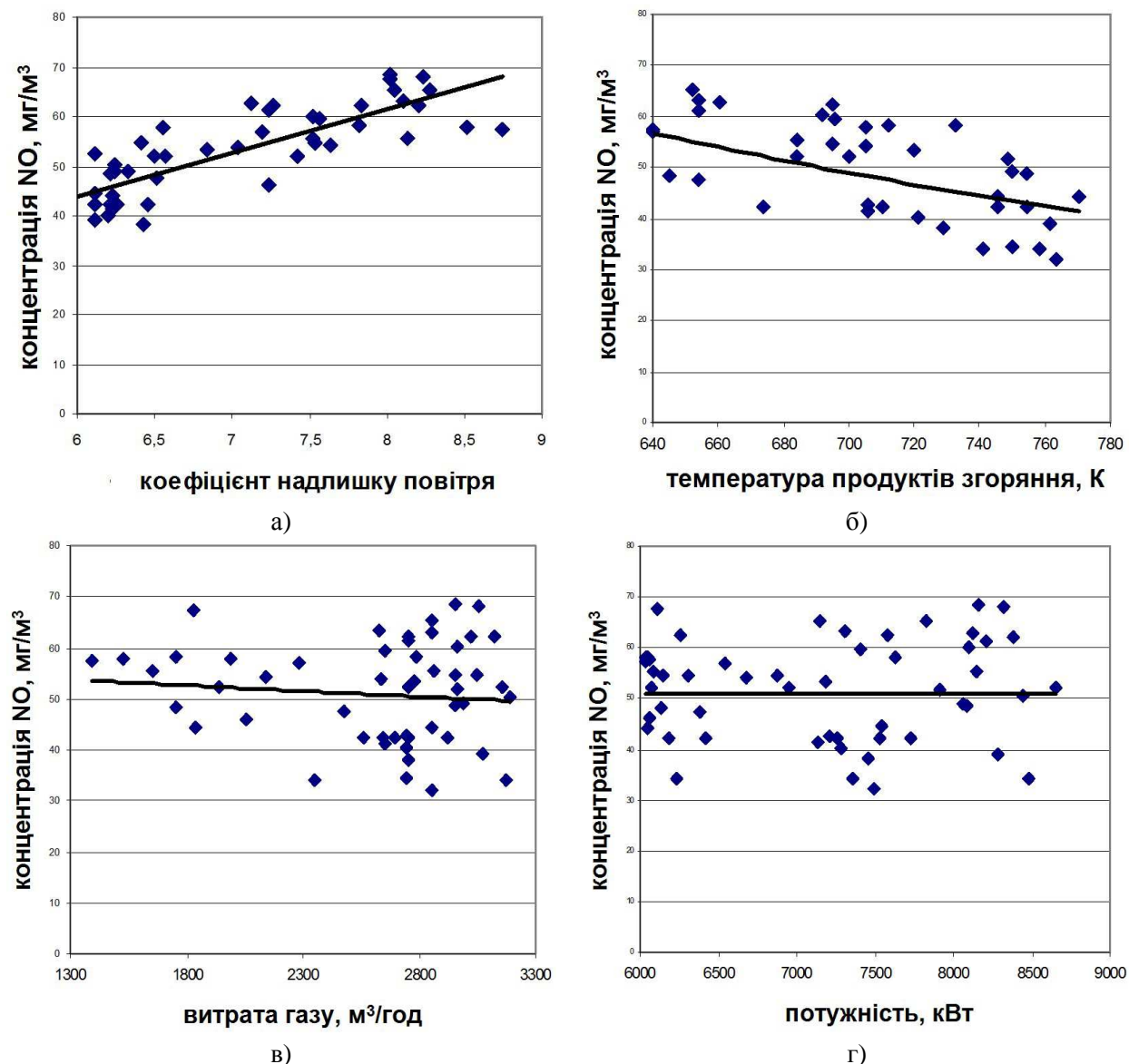
Рисунок 1 – Парний взаємозв'язок залежності концентрації оксиду азоту \text{NO} та надлишку повітря (а); температури продуктів згоряння (б); витрати газу (в); потужності (г)
