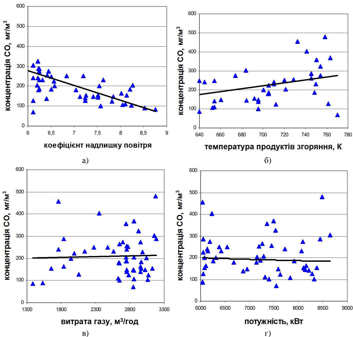
Рисунок 3 – Парний взаємозв’язок залежності концентрації оксиду вуглецю CO та надлишку повітря (а); температури продуктів згоряння (б); витрати газу (в); потужності (г)
