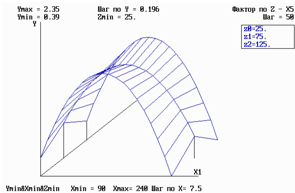
Рисунок 3 – Графік дослідження поверхні відгуку Y_1 = f(X_1, X_5) в тривимірному просторі при X_4=673 °K, X_6=2,5 МПа
