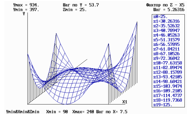
Рисунок 9 – Графіки частинних рівнянь регресії Y_3 = f(X_1, X_5) при X_2=137,5 Па, X_3=60\%Ar+40\%N_2 , X_4=773 °К
