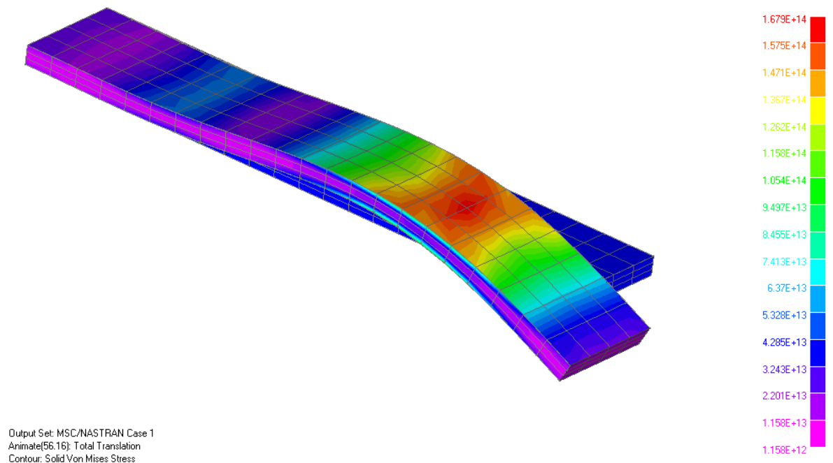
Рисунок 12 – Модель напружено-деформованого стану зміцненого зразка при мінімальному напруженні циклу, Па
