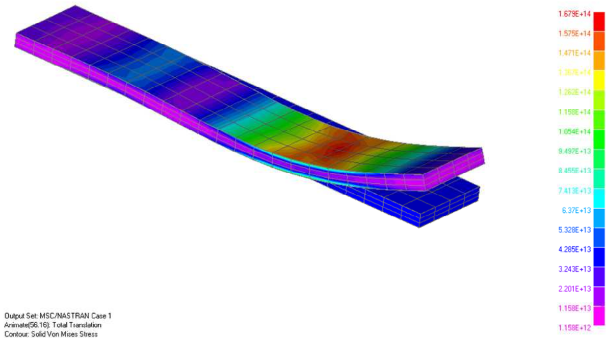
Рисунок 11 – Модель напружено-деформованого стану зміцненого зразка при максимальному напруженні циклу, Па
