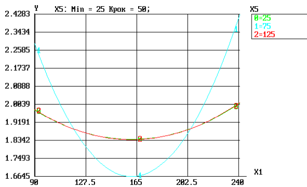
Рисунок 2 – Графіки частинних рівнянь регресії Y_1 = f(X_1, X_5) при X_3=60\%Ar+40\%N_2 , X_4=673 °K, X_6=2,5 МПа
