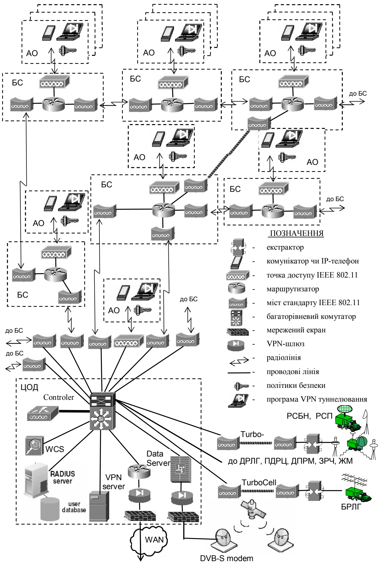
Рис. 1. Архітектура БМЗ авбр стандарту IEEE 802.11
