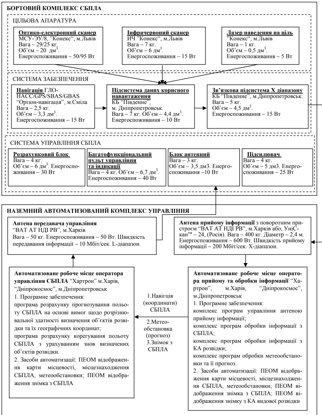
Рис. 2. Варіант структурної моделі автоматизованого комплексу добування інформації на базі стратегічного безпілотної літального апарата
