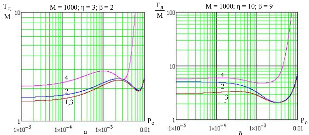
Рис. 2. Зависимость относительного среднего времени доставки сообщений от вероятности искажения единичного элемента в КС при: 1) m = 200 , P_{\hat{1}\hat{0}} = 0 ; 2) m = 200 , P_{\hat{1}\hat{0}} = 10^{-2} ; 3) m = 200 , P_{\hat{1}\hat{0}} = 10^{-5} ; 4) m = 500 , P_{\hat{1}\hat{0}} = 0
