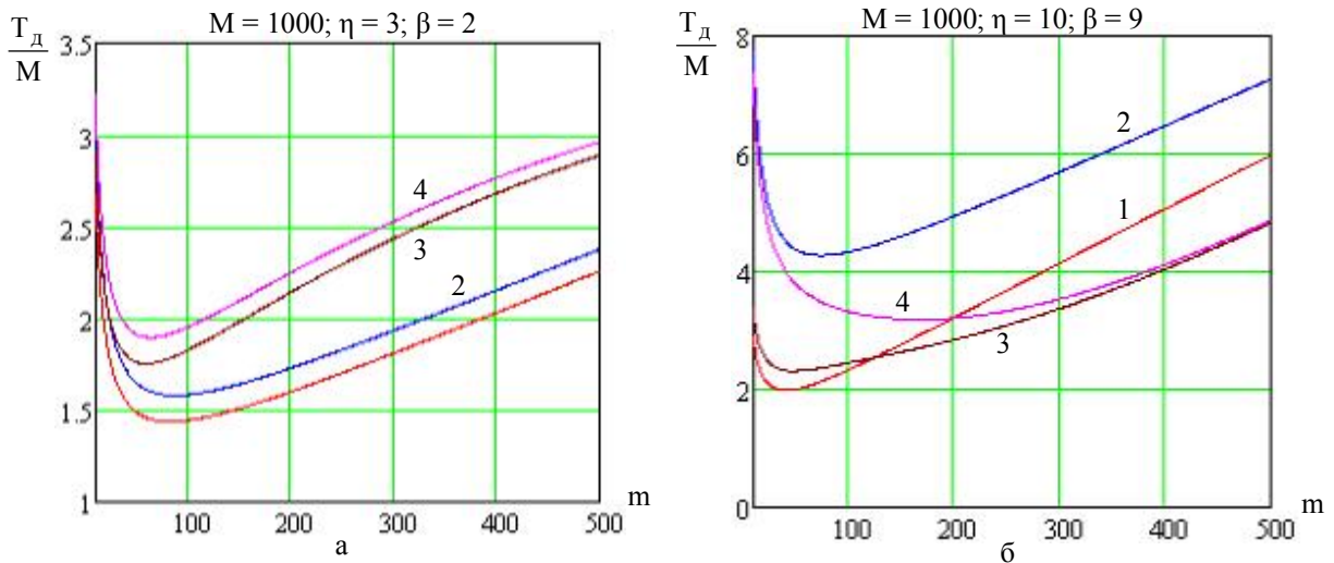
Рис. 1. Зависимость относительного среднего времени доставки сообщений от длины пакетов при: 1) P_0 = 10^{-4} , P_{\hat{1}\hat{0}} = 0 ; 2) P_0 = 10^{-4} , P_{\hat{1}\hat{0}} = 10^{-2} ; 3) P_0 = 10^{-3} , P_{\hat{1}\hat{0}} = 0 ; 4) P_0 = 10^{-3} , P_{\hat{1}\hat{0}} = 10^{-2}
