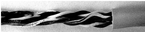
Рис. 9. Фотографія загальної деградації внутрішніх провідників і практично незшкодженої зовнішньої оболочці кабелю UTP5e, розміщеного в слабопровідному ґрунті, після впливу МЭМИ
