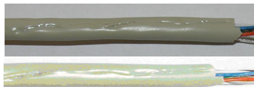
Рис. 12. Фотографії пошкодження зовнішньої ізоляційної оболочці кабелю UTP5e, розміщеного в слабопровідному ґрунті, після впливу МЭМИ
