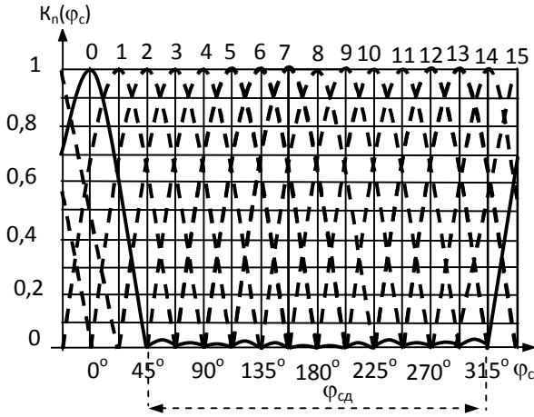
Рис. 1. Иллюстрация допуска доплеровского набег фаз \varphi_{сд} отраженных самолетом импульсов
