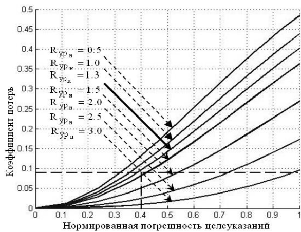
Рис. 1. Зависимость коэффициента потерь от погрешностей целеуказания
