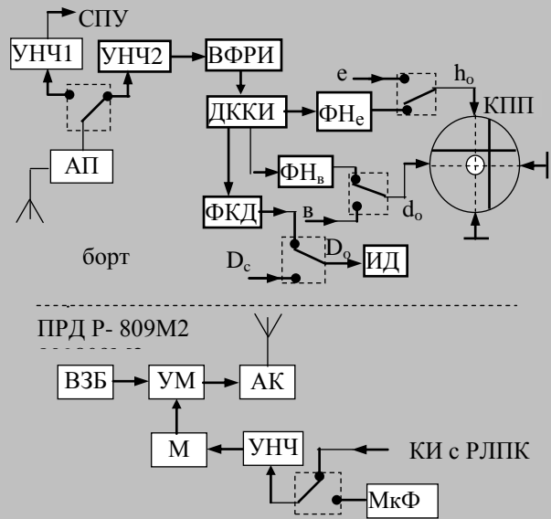
Рис. 2. Структурная схема КПСУ (вариант 1)
