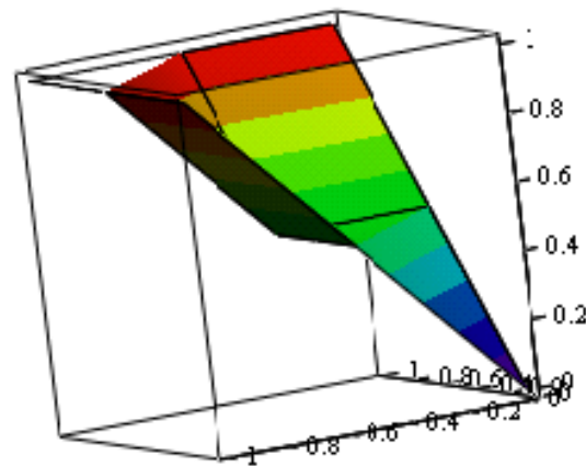
Рис. 4. Згортка нечітких змінних по правилу \max(x, y) .
