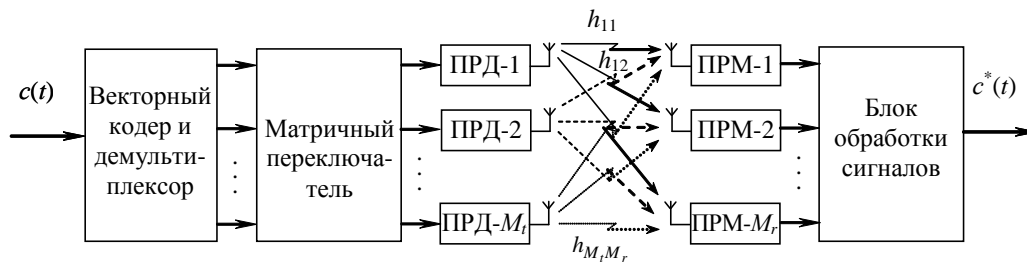
Рис. 1. Структурная схема ММО
