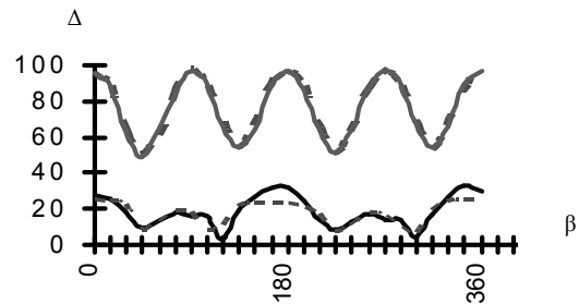
Рис. 2. Результати вимірів залежності параметра \Delta від значень кутів \beta для СПП-1 (дві верхні криві) і для СПП-2 (дві нижні криві)
