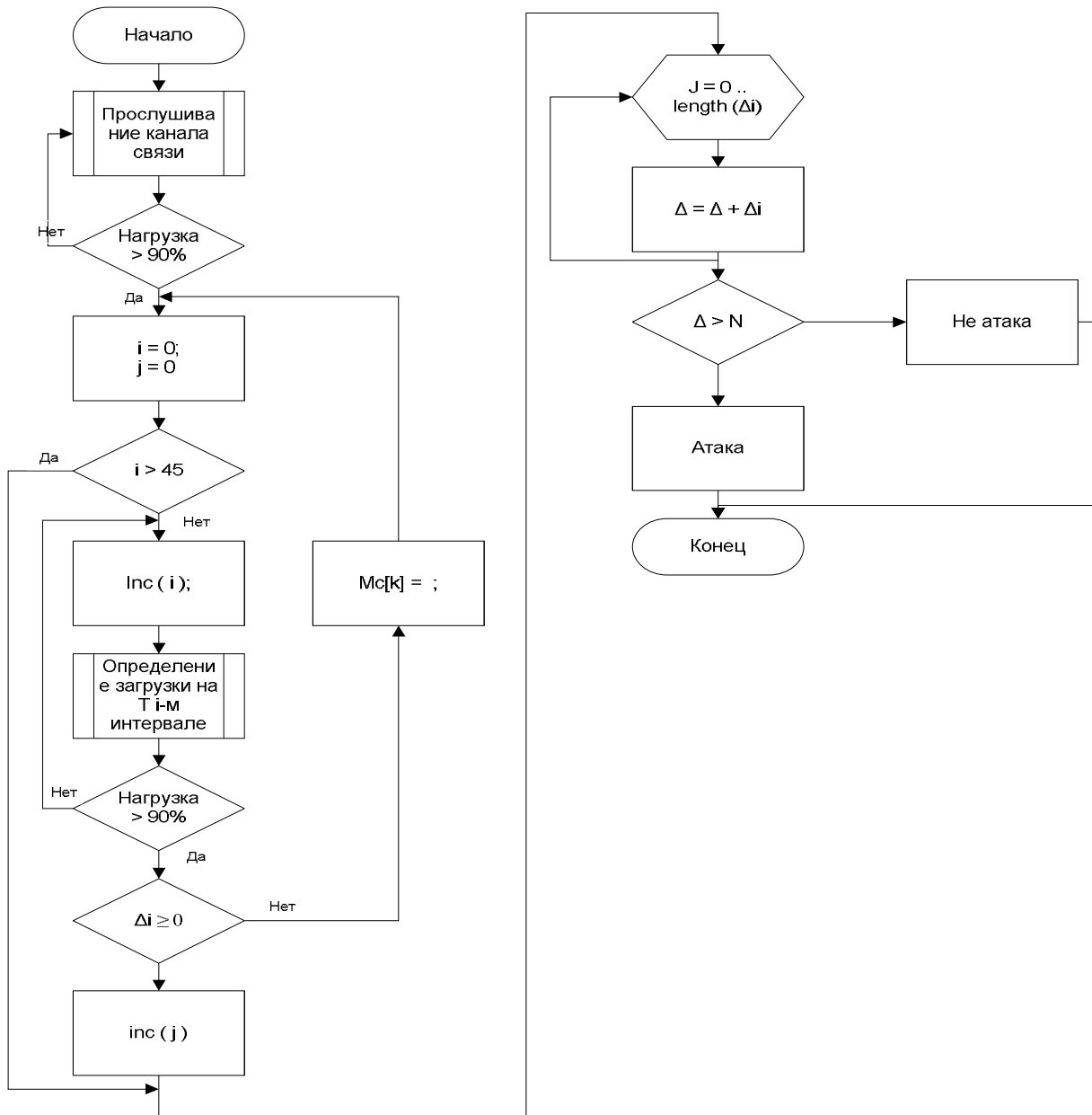
Рис. 2. Алгоритм обнаружения медленной DOS атаки
