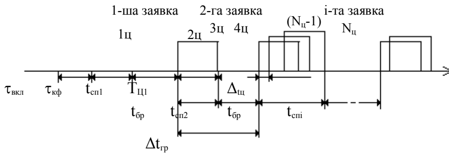
Рис. 1. Часова діаграма обстрілу цілей із складу типового нальоту ЗПН
