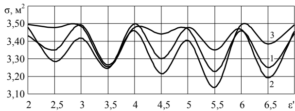
Рис. 4. Зависимость ЭПР модели №2 от относительной диэлектрической проницаемости сферической трехслойной оболочки (кривая 1 – d_{\text{внеш}} = 3 мм, кривая 2 – d_{\text{внеш}} = 5 мм, кривая 3 – d_{\text{внеш}} = 7 мм)
