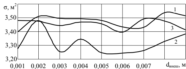
Рис. 5. Зависимость ЭПР модели №2 от толщины слоя сферической оболочки (кривая 1 – \epsilon' = 2 , кривая 2 – \epsilon' = 3,5 , кривая 3 – \epsilon' = 7 )
