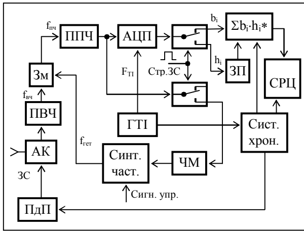
Рис. 8. Структура приймально-передавального тракту при формуванні квадратурних складових сигналу на проміжній частоті: ПдП – передавальний пристрій; ЗС – зондувальний сигнал; АК – антенний комутатор; ПВЧ (ППЧ) – підсилювач сигналів на високій (проміжній) частоті; Зм – змішувач; АЦП – аналого-цифровий перетворювач; \Sigma b_i \cdot h_i^* – пристрій обчислення згортки (узгоджений фільтр); СРЦ – система селекції рухомих цілей; ЗП – запам’ятовувачий пристрій; Стр.ЗС – строб зондувального сигналу; ГТІ – генератор тактових імпульсів; ЧМ – частотомір
