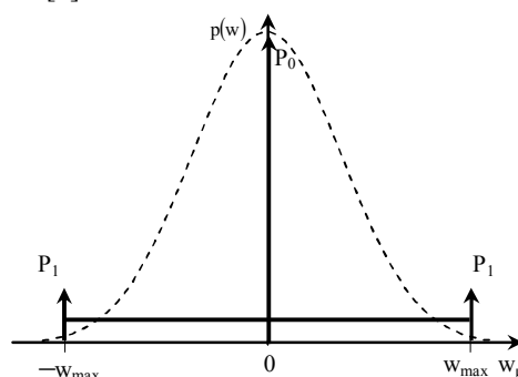
Рис. 1. Багатопікова щільність розподілу ймовірностей
