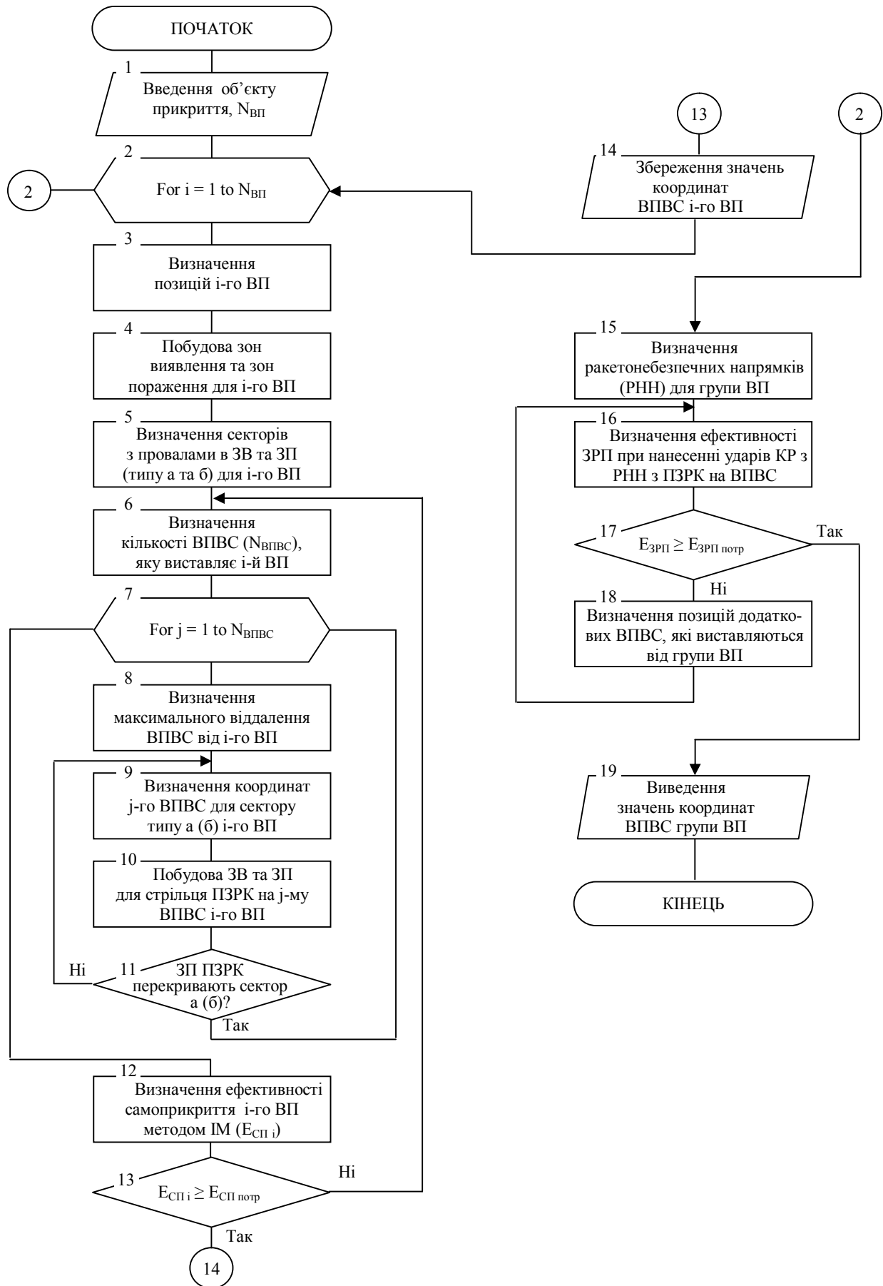
Рис. 1. Алгоритм вибору позицій для розміщення ВПВС з використанням моделей, реалізованих на основі геоінформаційної системи “Аргумент-2015”
