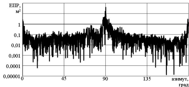
Рис. 6. ДЗВВ БпЛА "Орлан-10" для частоти зондування ССЦ 14,5 ГГц при куті місця зондування \epsilon_{\text{БпЛА}} = 5^\circ
