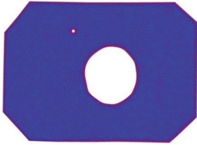
Рис. 4. Локалізований розряд, котрий має канал зниженої щільності. Вигляд із торця вакуумної камери
