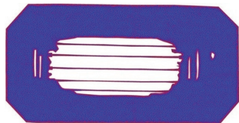
Рис. 3. Розряд із плазмою загального випромінювання. Вигляд через бічну циліндричну скляну прозору вакуумну камеру
