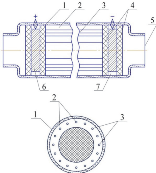
Рис. 2. Пристрій для отримання плазми загального від'ємного випромінювання великих розмірів:
