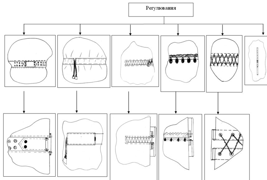
Рис.8. Трансформативні елементи принципу регулювання
