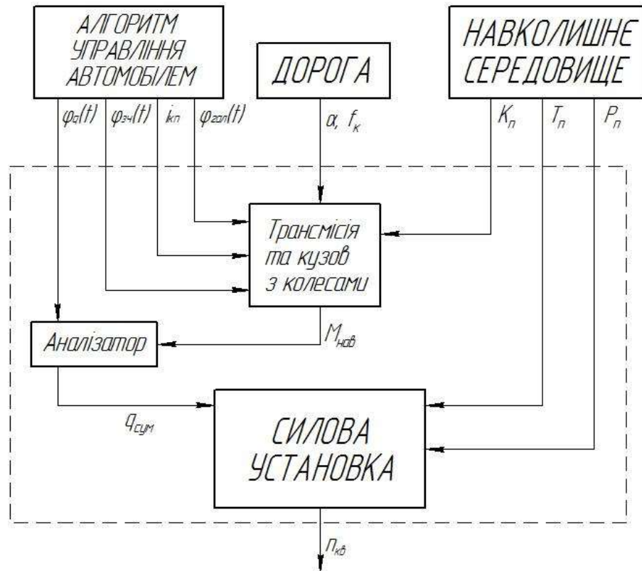
Рис. 1. Функціональна схема системи «Автомобіль з дизельним двигуном - дорога - навколишнє середовище»
