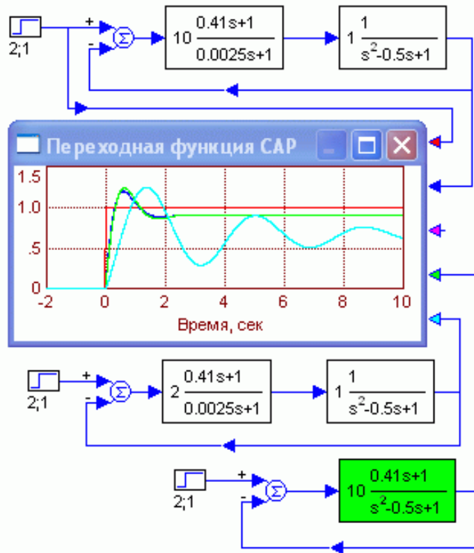
Рис. 1. Приклад моделювання САПР в PCM VisSim
