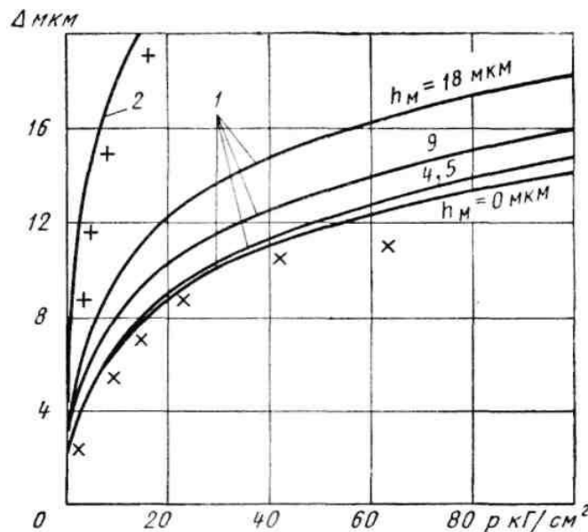
Рис. 1. Розрахункові криві впливу контактної сили на стикові деформації струганих поверхонь при: 1 - s = 0,28 ; 2 - s = 0,56 мм/дв.хід
