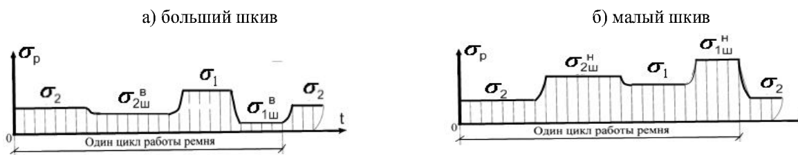
Рис. 2 – Циклы изменения напряжений в сечениях ремня
