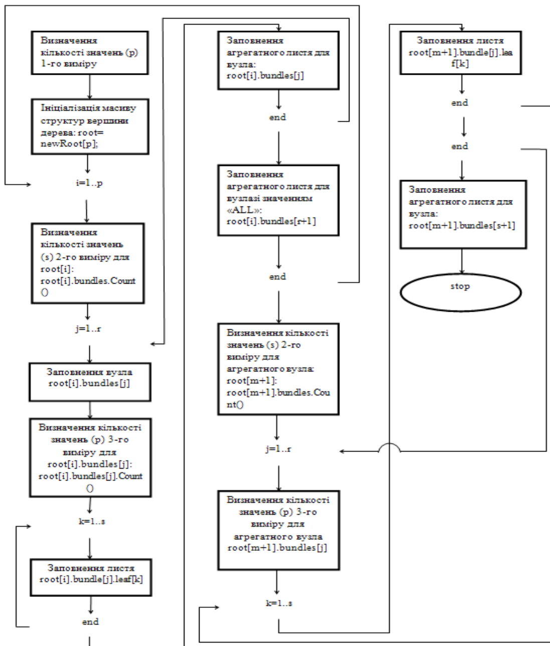
Рис. 4. Блок-схема алгоритму DWARF для куба з 3 вимірами
