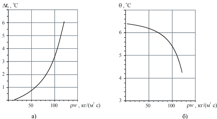
Рис. 4. Падение температуры кипения \Delta t_0 хладагента R142B (а) и температурные напоры \theta (б) в зависимости от массовой скорости \rho w хладагента R142B в испарителе при температурах кипения R142B t_0 = 0^\circ\text{C} , воды на входе t_{w1} = 8^\circ\text{C} и выходе t_{w2} = 5^\circ\text{C} из испарителя
