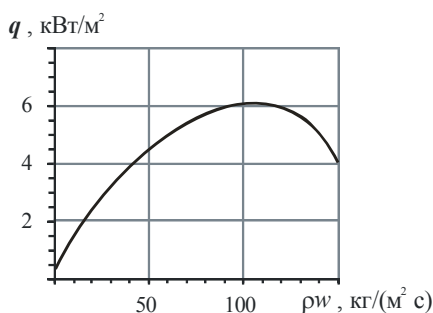
Рис. 5. Плотности теплового потока q в зависимости от массовой скорости \rho w хладагента R142B в испарителе при температурах кипения R142B t_0 = 0^\circ\text{C} , воды на входе t_{w1} = 8^\circ\text{C} и выходе t_{w2} = 5^\circ\text{C} из испарителя
