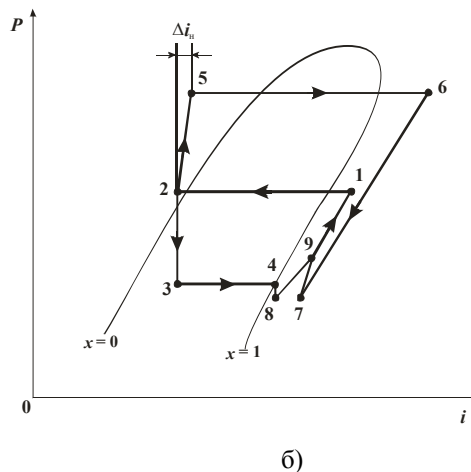
Рис. 1. Схема эжекторной ТУО (а) и цикл эжекторной холодильной машины (б), использующей теплоту уходящих газов для охлаждения воздуха на входе дизеля: Г – генератор паров НРТ; Э – эжектор; Кн – конденсатор НРТ; Н – насос НРТ; ДК – дроссельный клапан; НВ – наружный воздух; И-ВО – испаритель НРТ-воздухоохладитель; ОНВ – охладитель наддувочного воздуха водяной; К – компрессор; УТ – утилизирующая турбина
