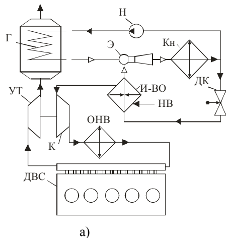
Рис. 1. Схема эжекторной ТУО (а) и цикл эжекторной холодильной машины (б), использующей теплоту уходящих газов для охлаждения воздуха на входе дизеля: Г – генератор паров НРТ; Э – эжектор; Кн – конденсатор НРТ; Н – насос НРТ; ДК – дроссельный клапан; НВ – наружный воздух; И-ВО – испаритель НРТ-воздухоохладитель; ОНВ – охладитель наддувочного воздуха водяной; К – компрессор; УТ – утилизирующая турбина
