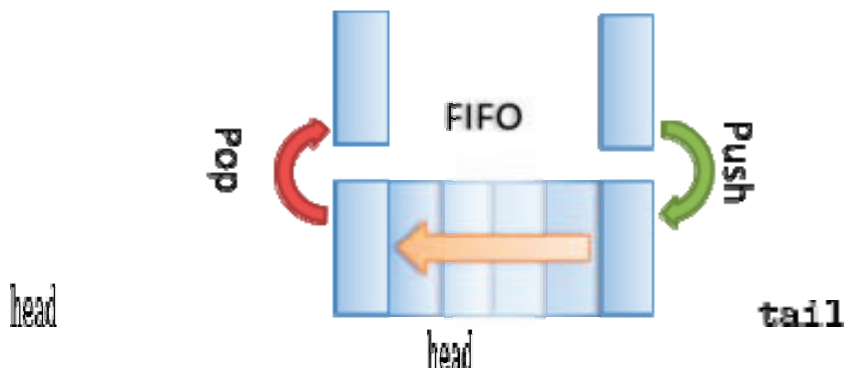
Рис. 1. Побудова черги
