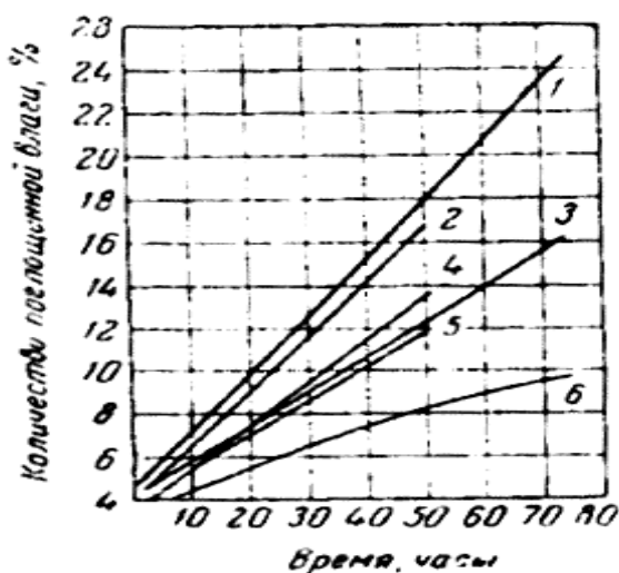
Рис. 1. Влияние добавок на скорость поглощения влаги аммиачной селитрой: 1 — без добавок; 2 — 0,5–1,0% смолистого мазута; 3 — 0,5% парафина; 4 — 0,5% смолы, битума, вазелина и парафина; 5 — 0,5% парафинистого мазута; 6 — 1% парафинистого мазута
