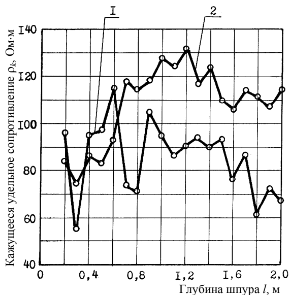
Рис. 3. Характерные зависимости кажущегося удельного сопротивления от расстояния к контуру горизонтальной выработки
