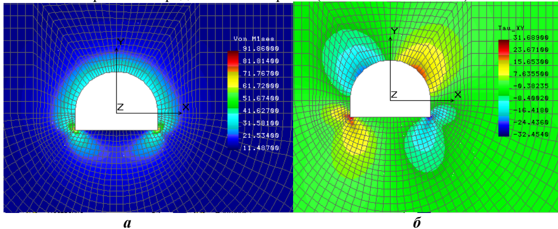
Рис. 1. Картины распределения эквивалентных и касательных напряжений (этап без пропила)
