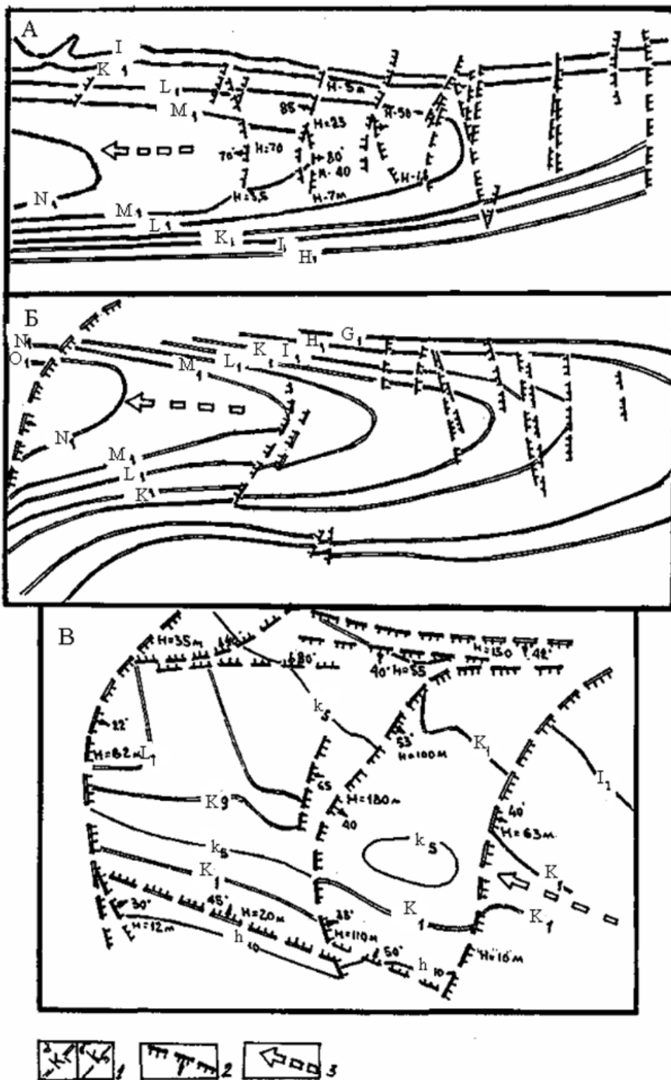
Рис.1. Схематические геологические разрезы: А — Боково-Хрустальской, Б — Чистяково-Снежнянской, В — Ряснянской синклинали: 1 — маркирующие горизонты: а — известняки, б — угли; 2 — тектонические разрывы; 3 — направление перемещения материала при складкообразовании
