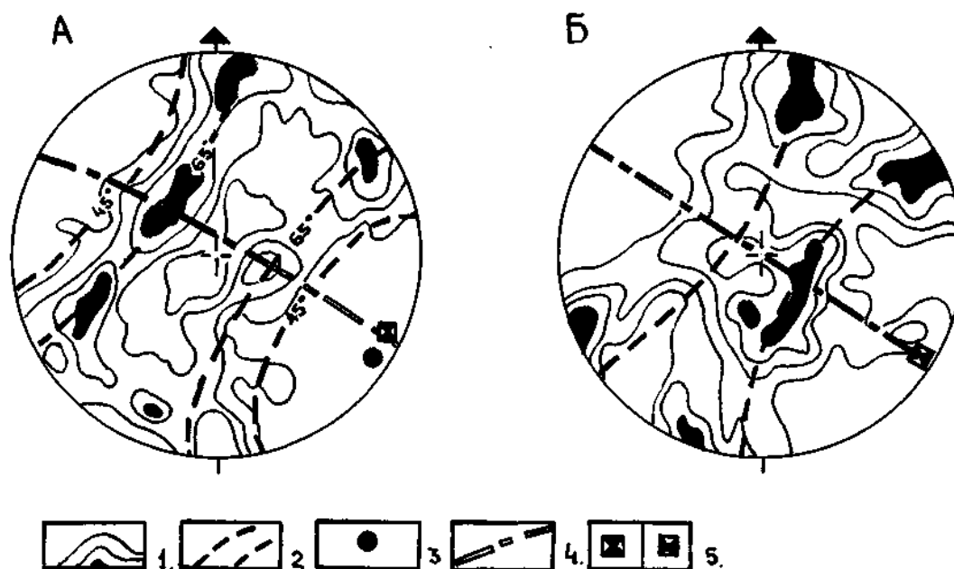
Рис.2. Сводные стереограммы полюсов трещин со «струйчатостью»: А — Донецко-Макеевский район, Б — Центральный район (по В.В.Эзу, 1962): 1 — изолинии плотности полюсов трещин; 2 — следы конических поверхностей; 3 — оси симметрии; 4 — осевые плоскости складок; 5 — шарниры складок: а — Ряснянской синклинали, б — Главной антиклинали
