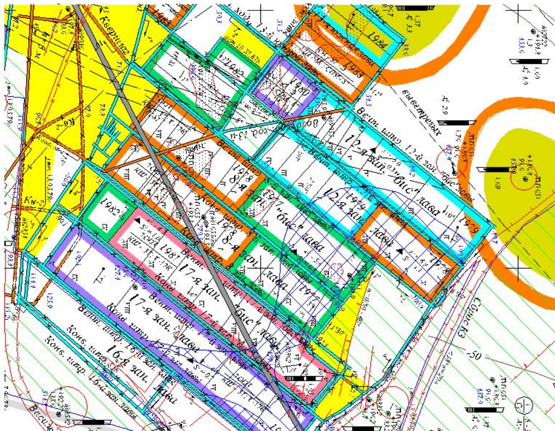
Рис. 2. Вкопювання з плану гірничих робіт пласта С 11 шахти «Южнодонецкая № 1»
