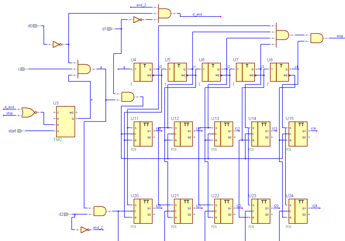
Рис. 1. Принципиальная схема цифрового осциллографа
